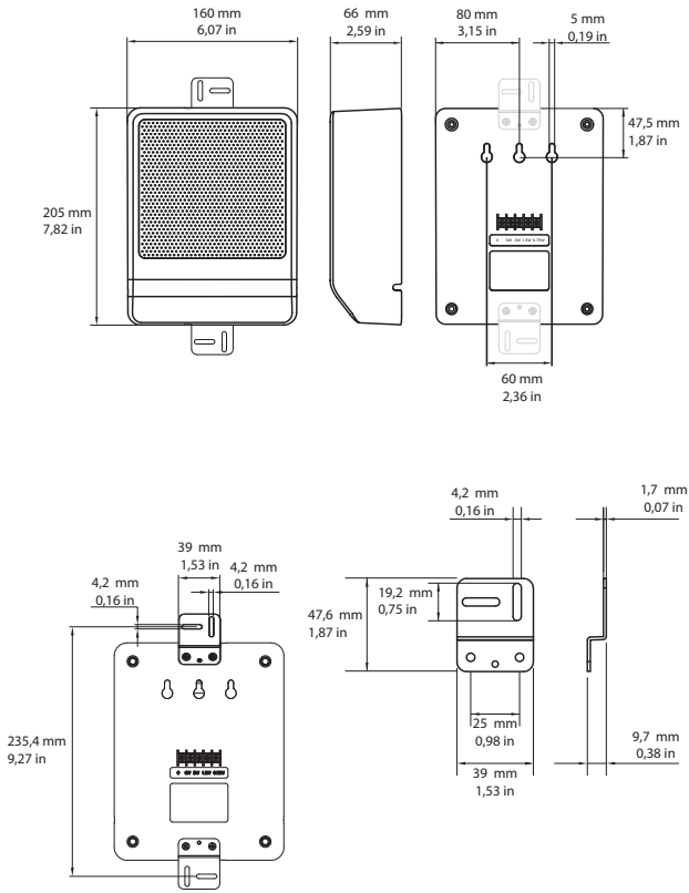
Размеры LB10-UC06-Fx
