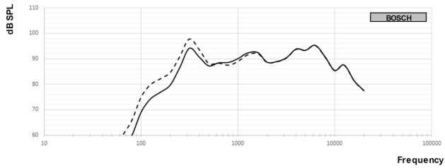
Частотная характеристика — Результат полношагового измерения - - - Результат полушагового измерения
